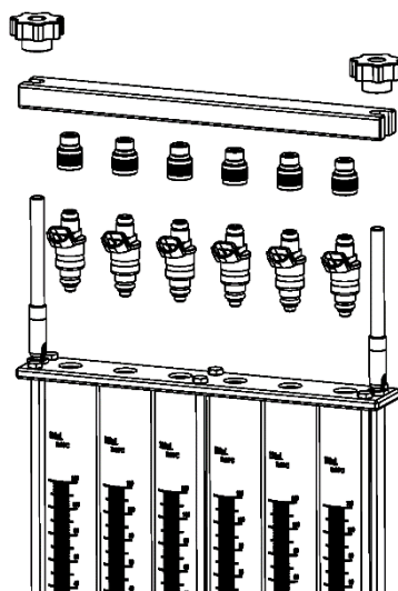
(Установка форсунок с верхней подачей топлива)
